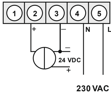
M1-1/3/6 in Verbindung mit einem 3-Leiter-Sensor 0/4-20 mA
