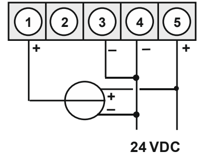
M1-1/3/6/7 in Verbindung mit einem 3-Leiter-Sensor 0-10 V
