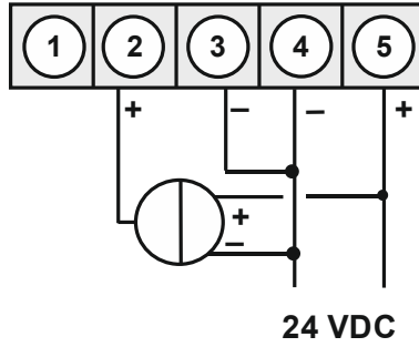
M1-1/3/6/7 in Verbindung mit einem 3-Leiter-Sensor 0/4-20 mA
