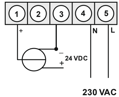
M1-1/3/6 in Verbindung mit einem 3-Leiter-Sensor 0-10 V
