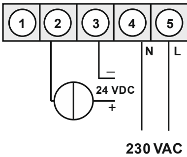
M1-1/3/6 in Verbindung mit einem 2-Leiter-Sensor 4-20 mA
