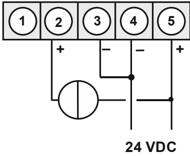
M1-1/3/6/7 in Verbindung mit einem 2-Leiter-Sensor 4-20 mA
